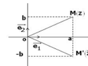
M(\bar{z}) و M(z) متماثلان بالنسبة للمحور الحقيقي
